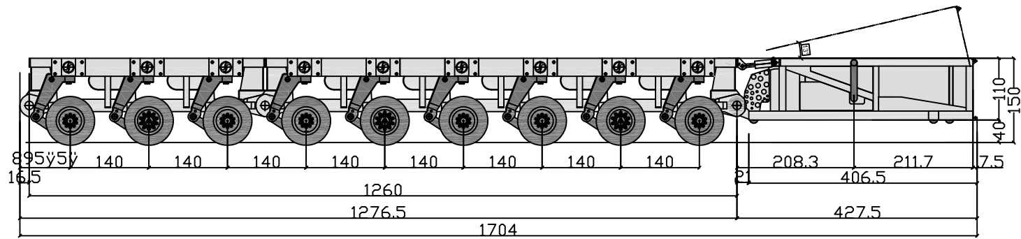
Seitenansicht
