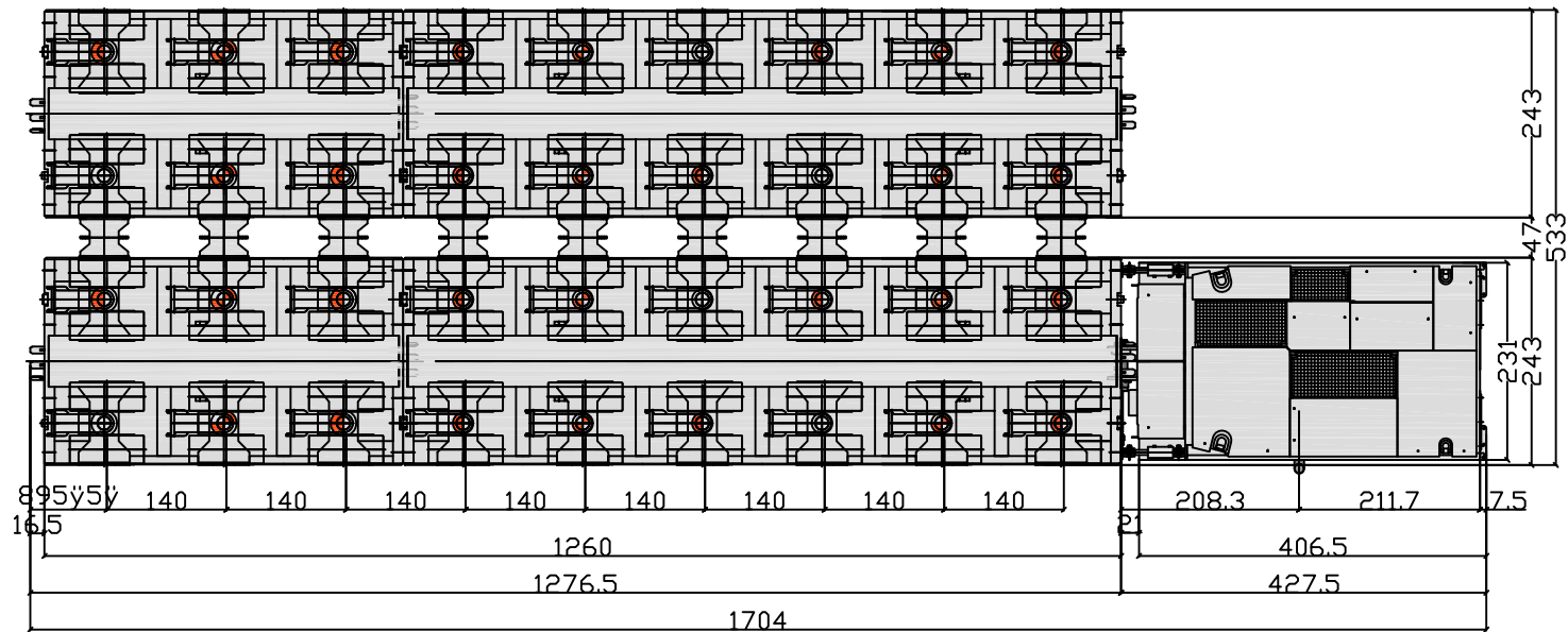
Draufsicht
