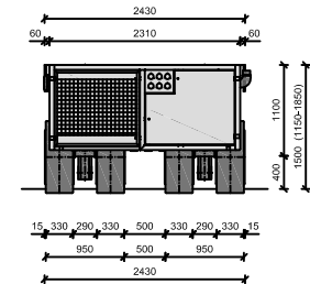
Frontansicht
