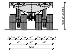
Frontansicht
