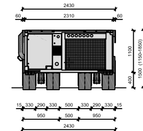
Frontansicht
