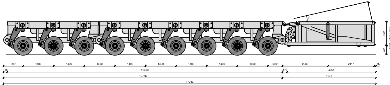
Seitenansicht
